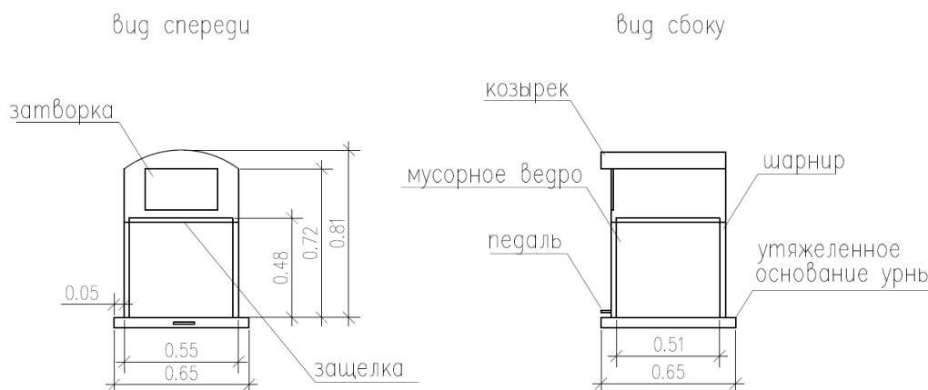
Рисунок 2. Проект урны для раздельного сбора отходов
