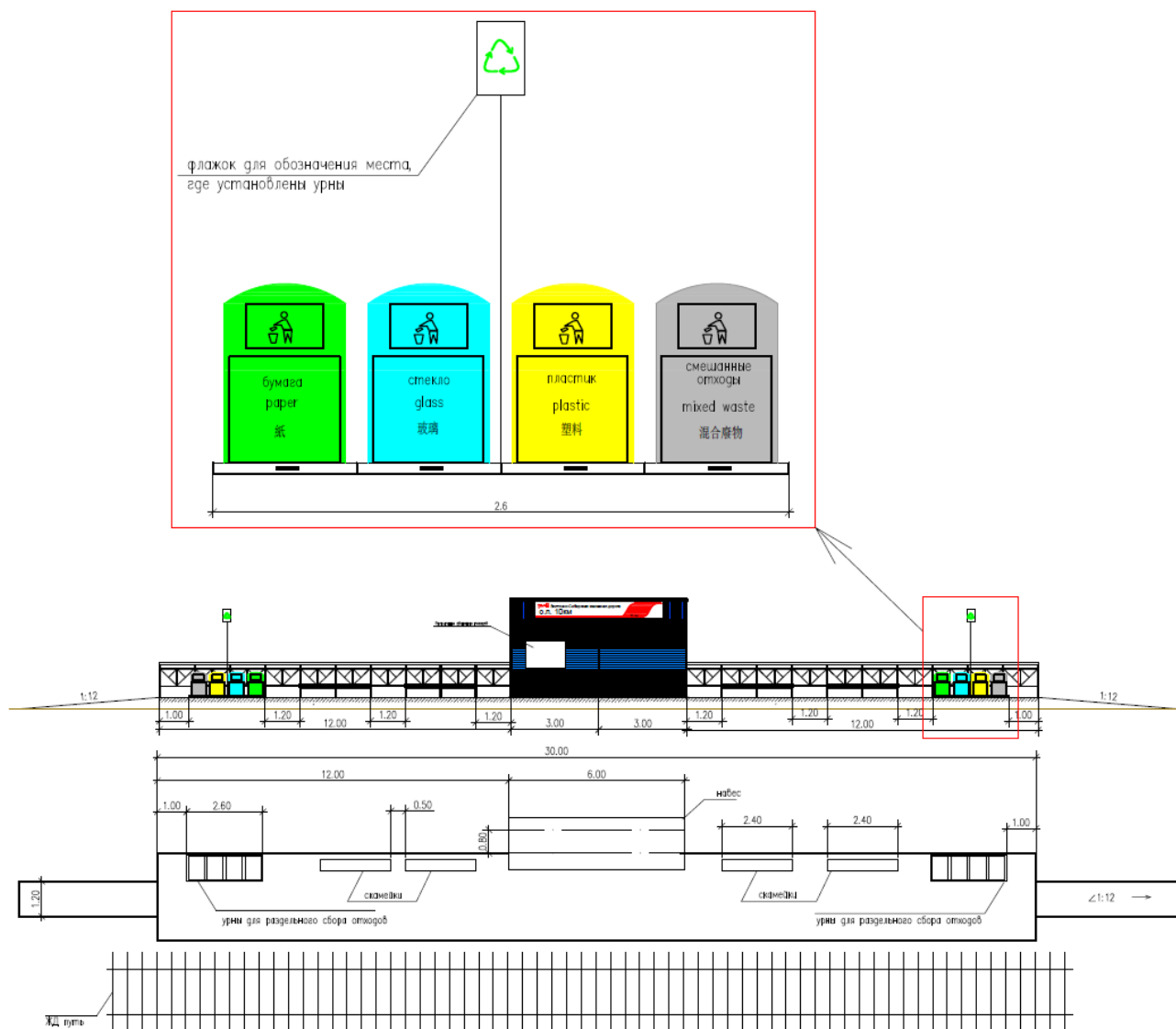
Рисунок 3. Проект платформы с урнами для раздельного сбора отходов
